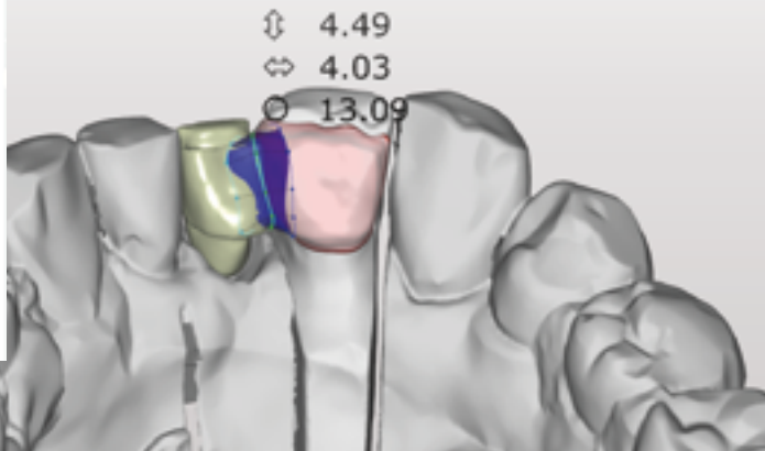
Abb. 27 (oben) Digitale Konstruktion des Zirkonoxidkeramikgerüsts (Zahn-technik und Bild: ZTM Tomonari Okawa, Hamburg)
